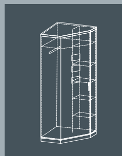
Шкаф угловой Д931xГ931xВ2264
