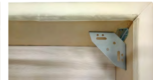
Усиленные уголки-держатели основания
